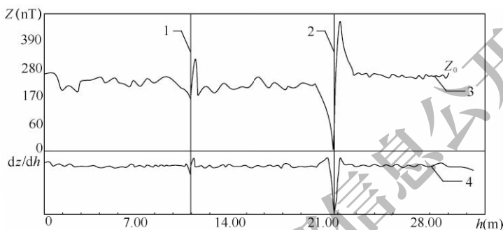
图 9.4.1 磁场垂直分量 (Z)
